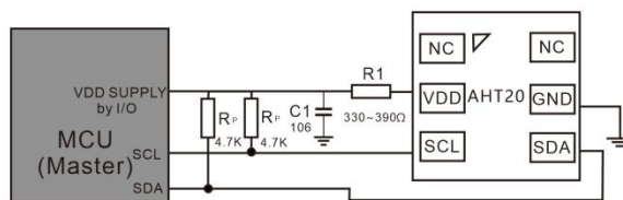
图15 典型应用电路。
